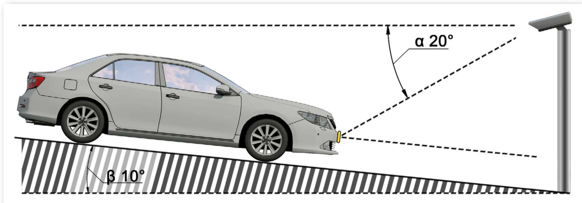
Рисунок 9 — Размещение камеры для видеонаблюдения дороги с уклоном
