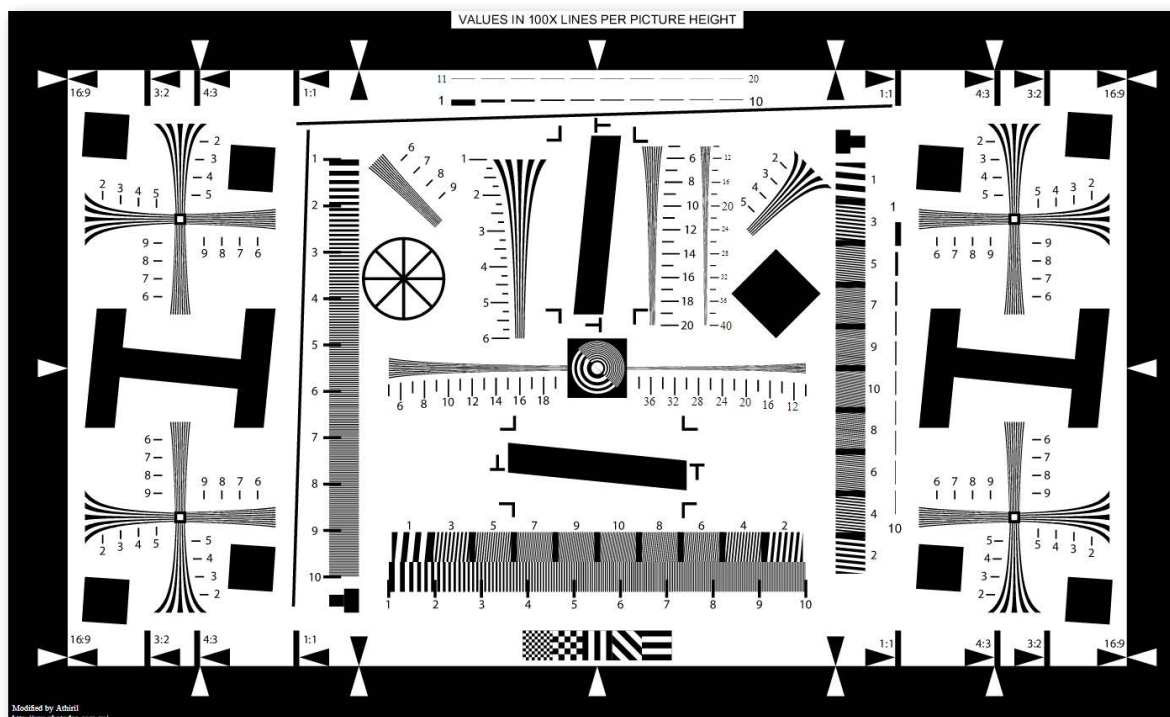
Рисунок 5 — Пример тестовой таблицы (согласно стандарту ISO 12233)
