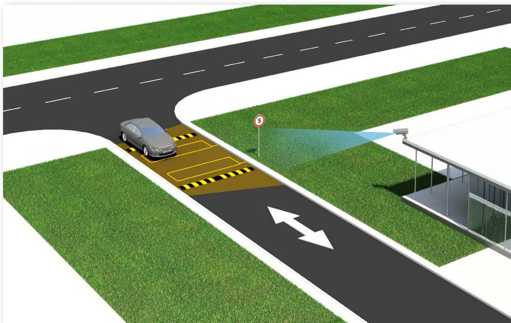
Рисунок 13 — Размещение камеры на нерегулируемом контрольно-пропускном пункте с двусторонним движением
