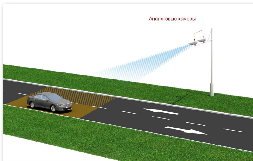
Рисунок 14 — Размещение аналоговых камер у края автотрассы на Г-образной опоре
