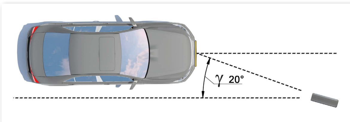
Рисунок 8 — Максимальный угол установки камеры по горизонтали
